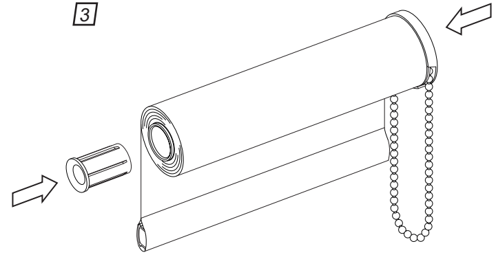
Schieben Sie das Bedien- und Montageprofil in die Rollowelle. Sie können die Bedienseite dabei selbst festlegen.
